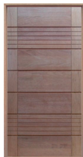
PORTA PIVOTANTE BBB-R 8 FRISOS MONTADA NO BATENTE CAIXA 14 E COM PIVÔ CÓDIGO 1520 - 2,10m x 0,90m - Final: 2,15m x 0,98m CÓDIGO 1521 - 2,10m x 1,00m - Final: 2,15m x 1,08m CÓDIGO 1522 - 2,10m x 1,10m - Final: 2,15m x 1,18m CÓDIGO 1523 - 2,10m x 1,20m - Final: 2,15m x 1,28m
