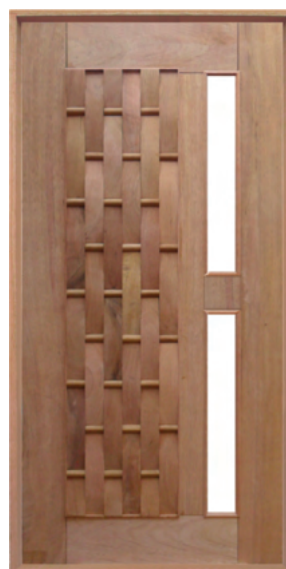
PORTA PIVOTANTE COURO LONGO VIDRO MONTADA NO BATENTE CAIXA 14 E COM PIVÔ CÓDIGO 1580 - 2,10m x 0,90m - Final: 2,15m x 0,98m CÓDIGO 1581 - 2,10m x 1,00m - Final: 2,15m x 1,08m CÓDIGO 1582 - 2,10m x 1,10m - Final: 2,15m x 1,18m CÓDIGO 1583 - 2,10m x 1,20m - Final: 2,15m x 1,28m
