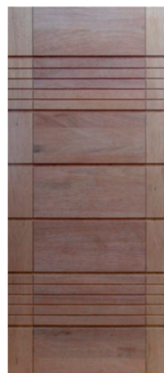
PORTA PIVOTANTE BBB-R 8 FRISOS CÓDIGO 2035 - 2,10m x 0,62m CÓDIGO 2036 - 2,10m x 0,72m CÓDIGO 2037 - 2,10m x 0,82m CÓDIGO 2038 - 2,10m x 0,92m CÓDIGO 2039 - 2,10m x 1,02m CÓDIGO 2040 - 2,10m x 1,12m CÓDIGO 2041 - 2,10m x 1,22m
