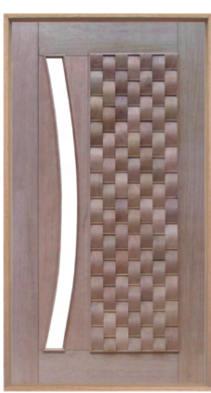
PORTA PIVOTANTE COURO VIDRO EM ARCO MONTADA NO BATENTE CAIXA 14 E COM PIVÔ CÓDIGO 1572 - 2,10m x 0,90m - Final: 2,15m x 0,98m CÓDIGO 1573 - 2,10m x 1,00m - Final: 2,15m x 1,08m CÓDIGO 1574 - 2,10m x 1,10m - Final: 2,15m x 1,18m CÓDIGO 1575 - 2,10m x 1,20m - Final: 2,15m x 1,28m
