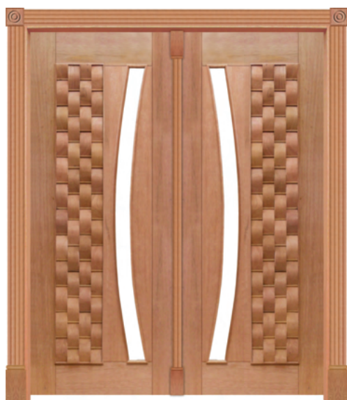
PORTAL PIVOTANTE CASMAVI - 370 - COURO PARA VIDRO EM ARCO CÓDIGO 1150 - Portal com 2 folhas de 2,10m x 0,72m - Medida Final de 2,15m x 1,52m CÓDIGO 1151 - Portal com 2 folhas de 2,10m x 0,82m - Medida Final de 2,15m x 1,72m CÓDIGO 1152 - Portal com 2 folhas de 2,10m x 0,92m - Medida Final de 2,15m x 1,92m
