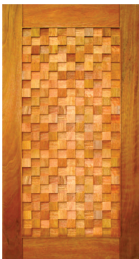
PORTA PIVOTANTE DETALHE CÓDIGO 2508 - 2,10m X 0,72m CÓDIGO 2509 - 2,10m X 0,82m CÓDIGO 2510 - 2,10m X 0,92m CÓDIGO 2511 - 2,10m X 1,02m CÓDIGO 2512 - 2,10m X 1,12m CÓDIGO 2513 - 2,10m X 1,22m
