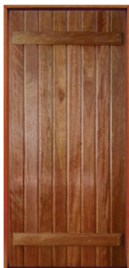
PORTA PIVOTANTE MEXICANA COM TRAVA EXTERNA MONTADA NO BATENTE CAIXA 14 E COM PIVÔ CÓDIGO 1536 - 2,10m x 0,90m - Final: 2,15m x 0,98m CÓDIGO 1537 - 2,10m x 1,00m - Final: 2,15m x 1,08m CÓDIGO 1538 - 2,10m x 1,10m - Final: 2,15m x 1,18m CÓDIGO 1539 - 2,10m x 1,20m - Final: 2,15m x 1,28m
