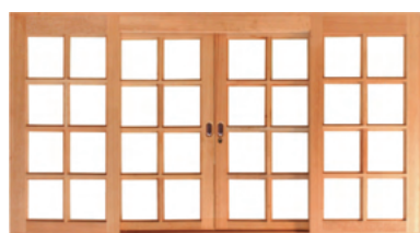
VITRÔ DE CORRER QUADRICULADO OU PANORÂMICO 4 FOLHAS RETO CÓDIGO 3086 - 1,10m x 2,40m ou CÓDIGO 3096 - 0,80m x 2,40m CÓDIGO 3087 - 1,10m x 2,00m ou CÓDIGO 3097 - 0,80m x 2,00m CÓDIGO 3088 - 1,10m x 1,80m ou CÓDIGO 3098 - 0,80m x 1,80m CÓDIGO 3089 - 1,10m x 1,60m ou CÓDIGO 3099 - 0,80m x 1,60m CÓDIGO 3090 - 1,10m x 1,40m ou CÓDIGO 3100 - 0,80m x 1,40m
