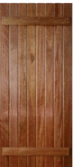
PORTA MEXICANA C/ TRAVA EXTERNA CÓDIGO 2417 - 2,10m x 0,62m CÓDIGO 2418 - 2,10m x 0,72m CÓDIGO 2419 - 2,10m x 0,82m CÓDIGO 2420 - 2,10m x 0,92m
