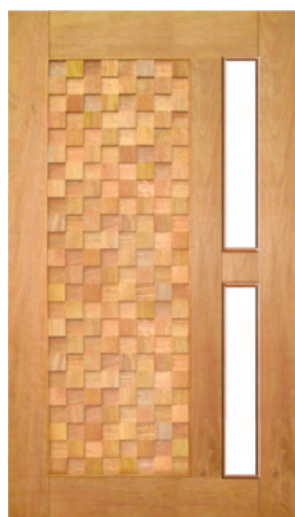
PORTA PIVOTANTE DETALHE PARA VIDRO CÓDIGO 2514 - 2,10m X 0,72m CÓDIGO 2515 - 2,10m X 0,82m CÓDIGO 2516 - 2,10m X 0,92m CÓDIGO 2517 - 2,10m X 1,02m CÓDIGO 2518 - 2,10m X 1,12m CÓDIGO 2519 - 2,10m X 1,22m
