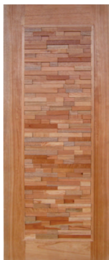
PORTA PIVOTANTE MIX CÓDIGO 2112 - 2,10m x 0,72m CÓDIGO 2113 - 2,10m x 0,82m CÓDIGO 2114 - 2,10m x 0,92m CÓDIGO 2115 - 2,10m x 1,02m CÓDIGO 2116 - 2,10m x 1,12m CÓDIGO 2117 - 2,10m x 1,22m
